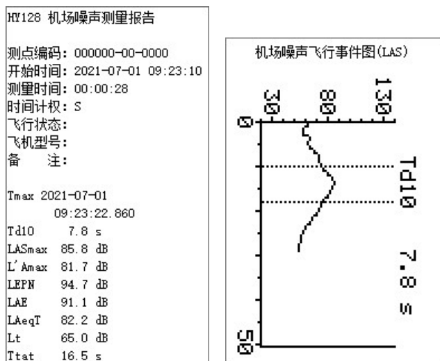
图 25 打印测量报告
