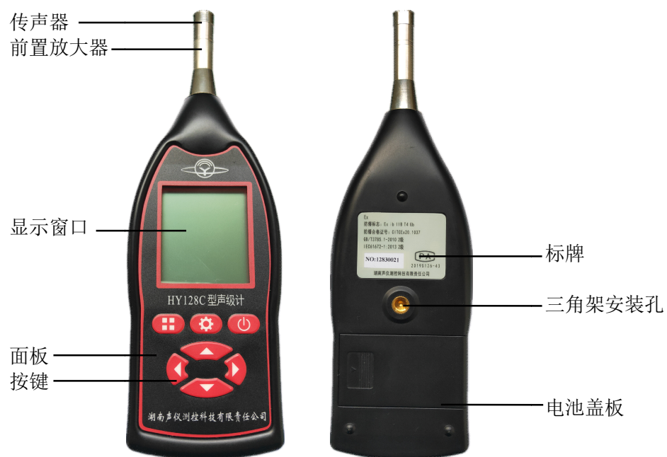
图 3 外形图
