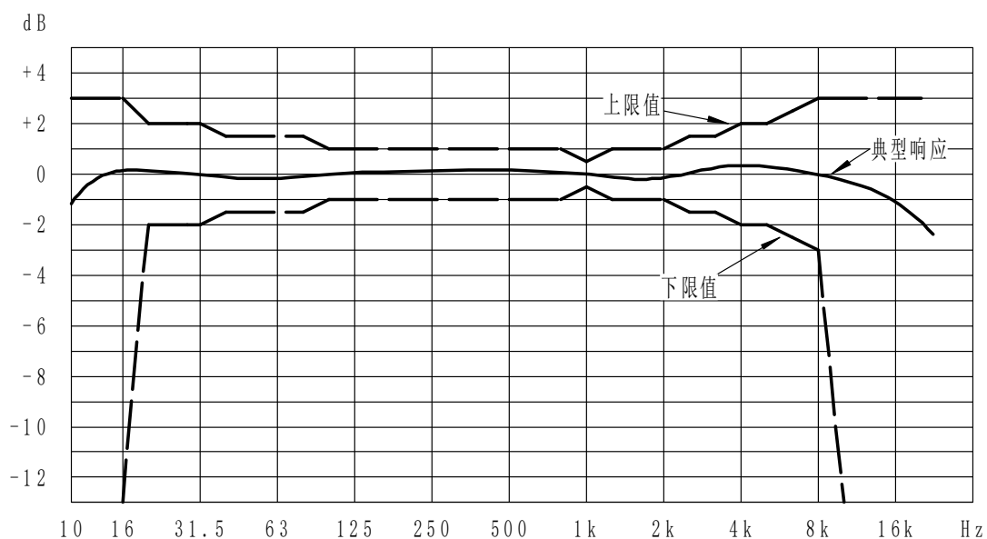
图 1 传声器的典型频率响应
