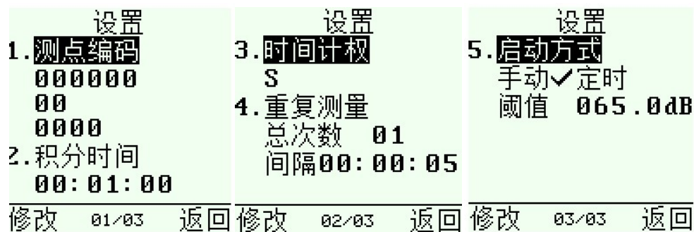
图 22 机场噪声设置界面
