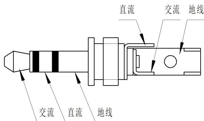
图 26 模拟输出插头的连接
