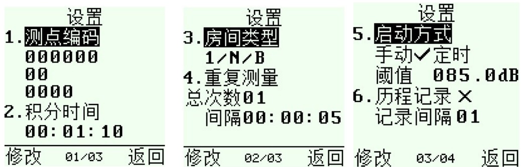
图 17 室内噪声界面中的设置
